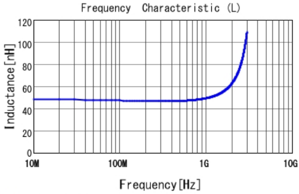
■ LQW15AN47NJ00 L
