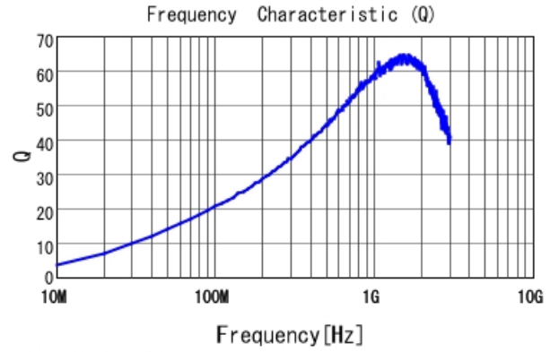
■ LQW15AN47NJ00 Q
