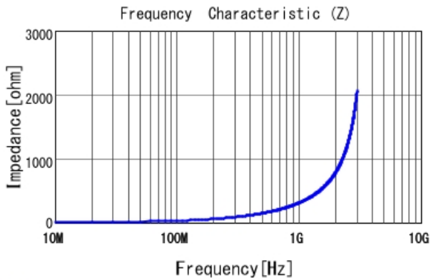
■ LQW15AN47NJ00 |Z|
