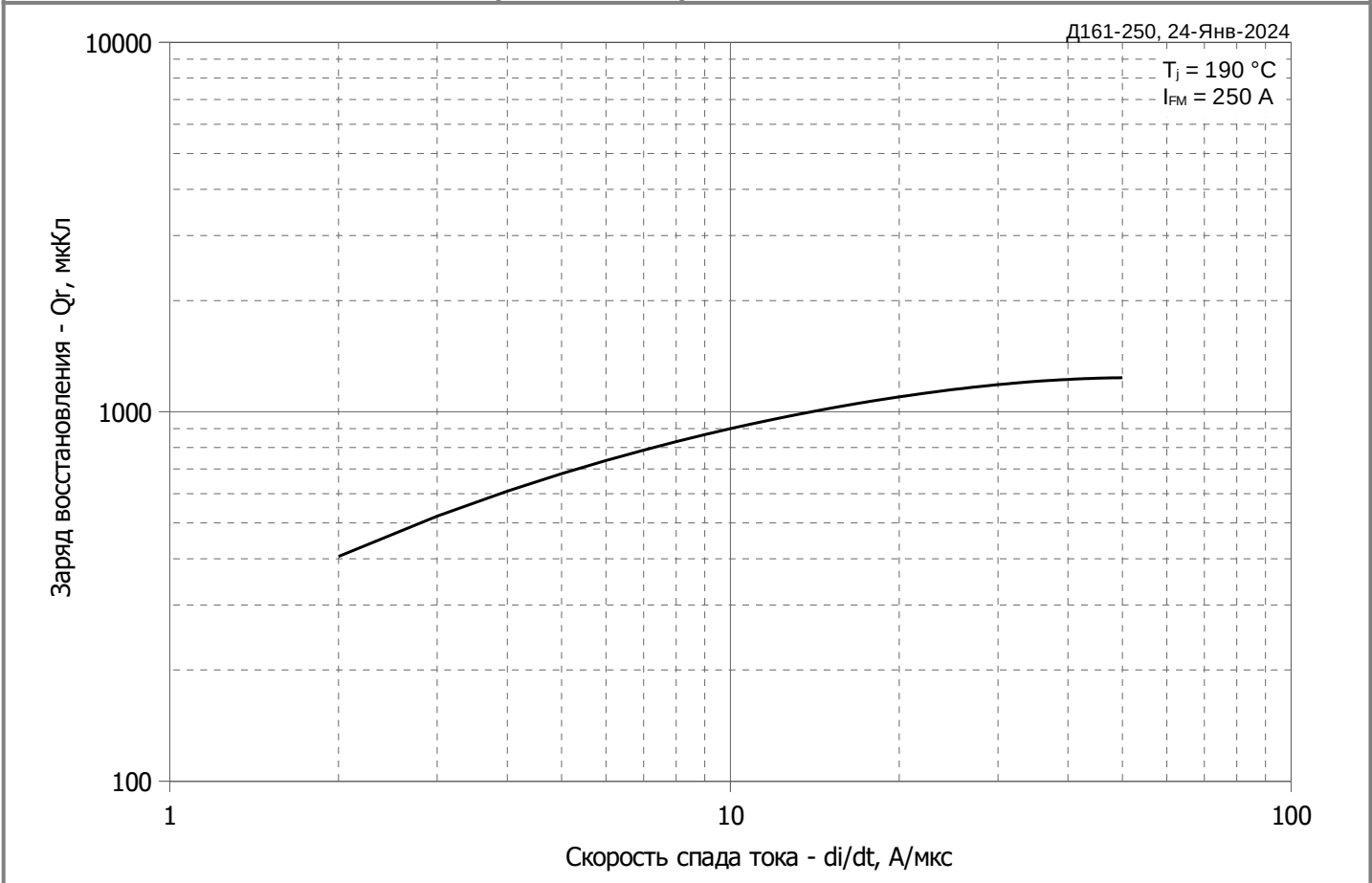
Рис. 4 – Зависимость максимального заряда обратного восстановления Q_{rr} от скорости спада прямого тока di_R/dt (по ГОСТ 24461, хорда 25%)
