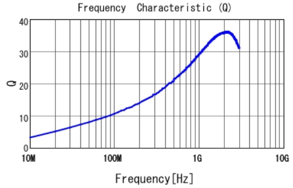
■ LQG15HS6N8G02 Q
