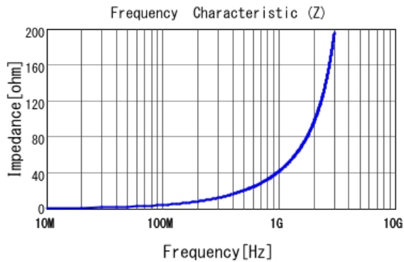
■ LQG15HS6N8G02 |Z|
