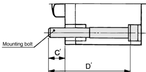
Rod side
