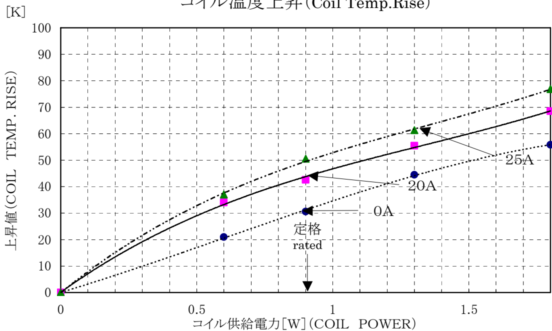
コイル温度上昇 (Coil Temp. Rise)
