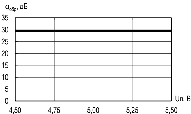
Зависимость обратной изоляции от напряжения питания ( f_{вх} = 2 \text{ ГГц} , P_{вх} = 0 \text{ дБм} )
