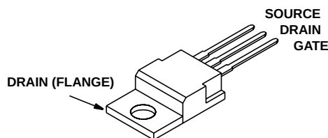
JEDEL TO-220AB
