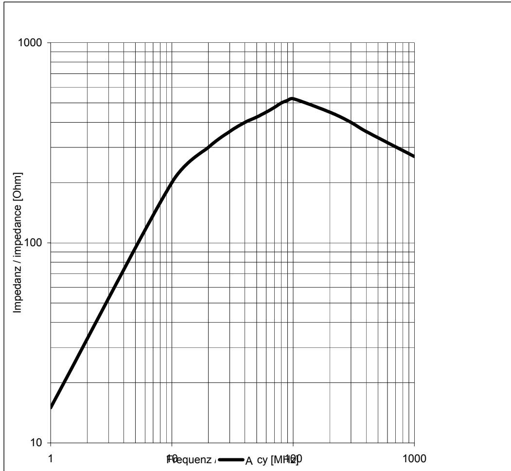
A: 3 Windungen / 3 turns
