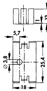
FK 213/SA-32 21 K/W
