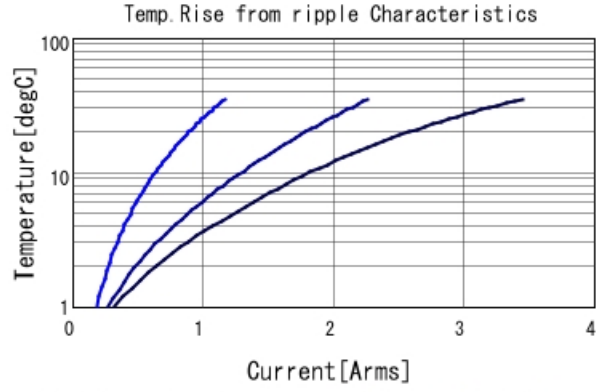
GRM55DR72E684KW01 Temp. rise ■ 30kHz ■ 100kHz ■ 300kHz
