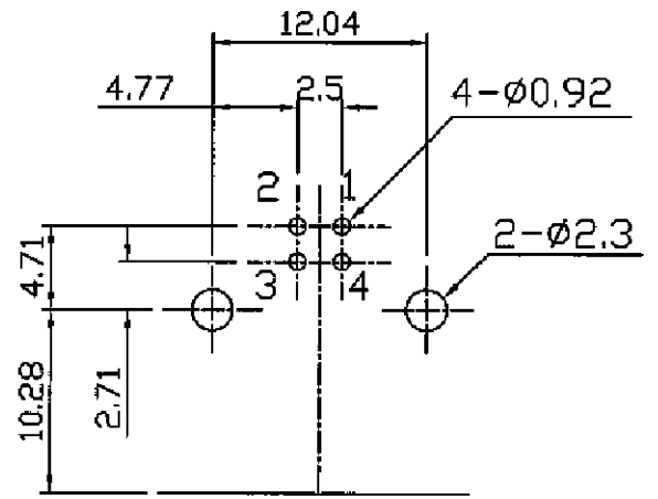
PCB EDGE (COMPONENT SIDE) PCB LAYOUT
