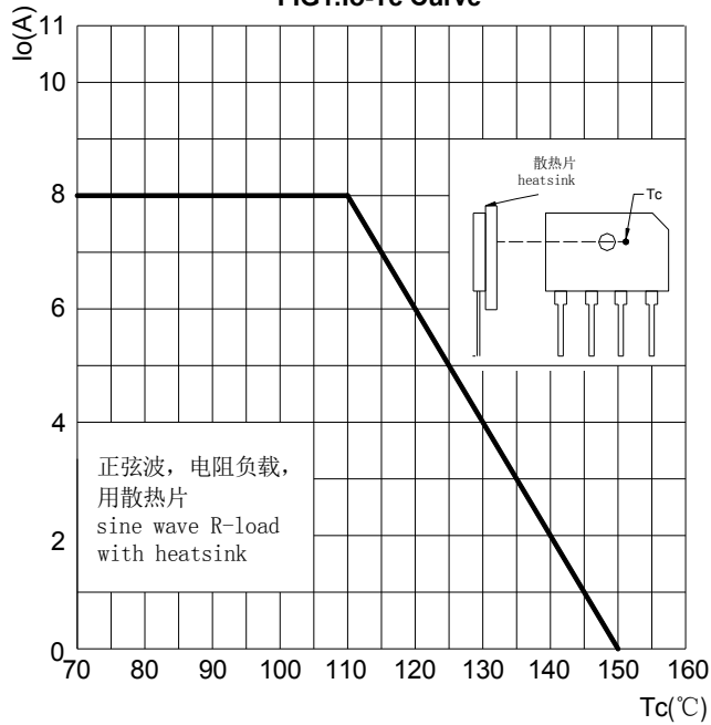
图1: I_o - T_c 曲线 FIG1: I_o - T_c Curve
