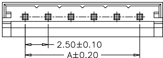
P.C.B LAYOUT
