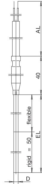
Type 902250/3x
