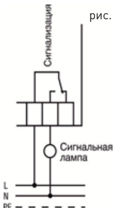
Рис. 16 Схема подключения цепи сигнализации.
