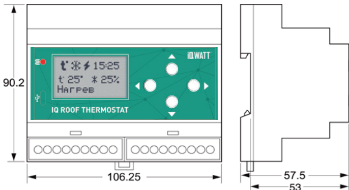
Рис. 1 Габаритные размеры модуля управления
