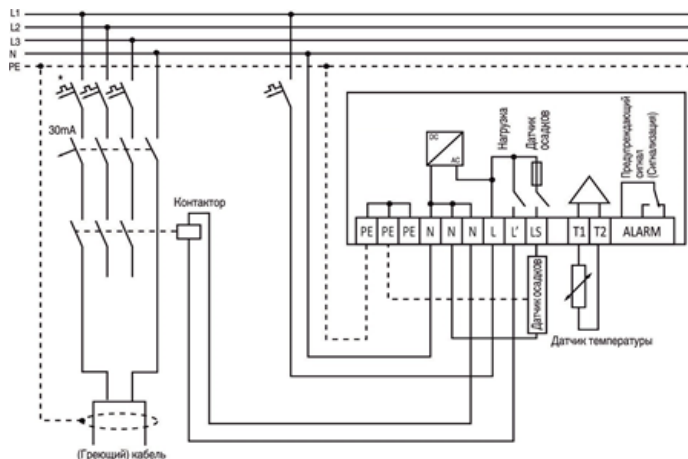
Рис. 15 Схема подключения греющего контура через контактор.
