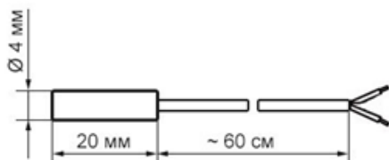
Рис. 2 Габариты датчика температуры
