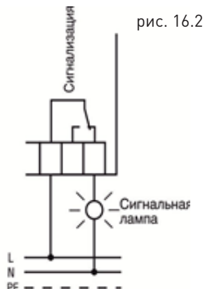
Рис. 16 Схема подключения цепи сигнализации.
