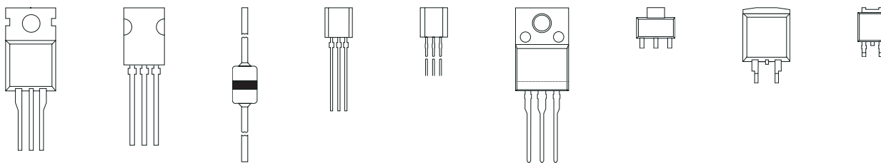
SOT-78 SOT-82 SOD-27 SOT-54 SOT-54B SOT-186A SOT-223 SOT-404 SOT-428
