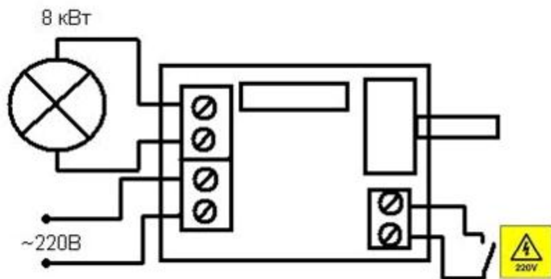
Схема подключения
