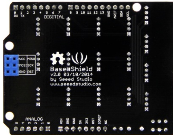
Base Shield v2 Back
