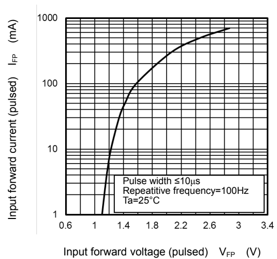
I_{FP} - V_{FP}
