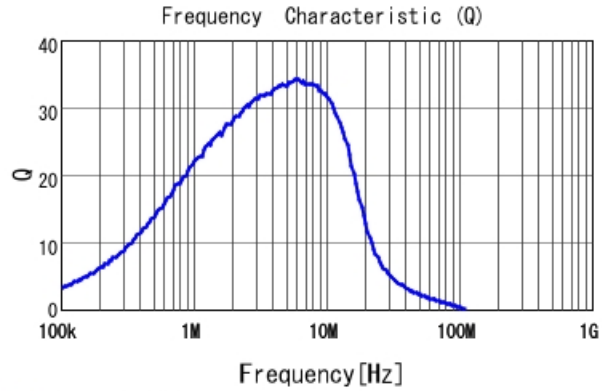
■ LQM21PN1R0MC0 Q
