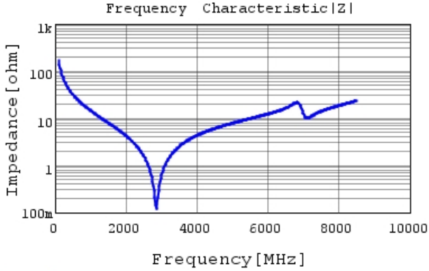
GCQ1555C1H9R7BB01 |Z| DC0V, 25degC
