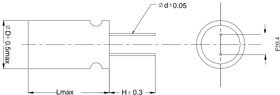
Fig. 2 Dimension
