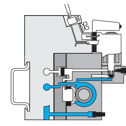
4/2 bistable module
