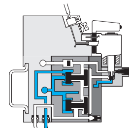
4/2 monostable module
