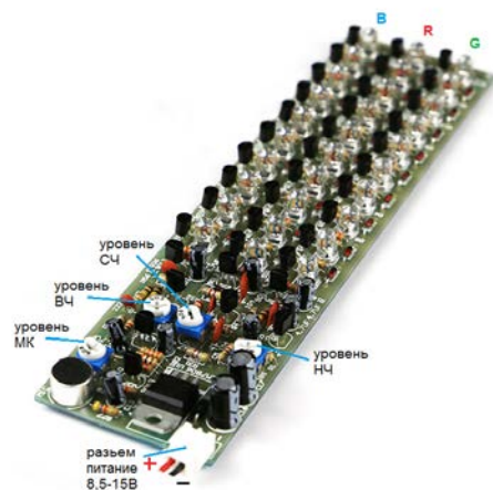
Эскиз подключения
