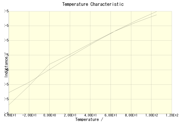
SLF12575T-470M2R7-PF(DC = 0A) SLF12575T-470M2R7-PF(DC = 1.35A)
