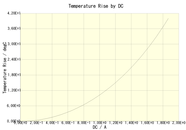
SLF10145T-470M1R4-PF(Amb. Temp. = 20degc)
