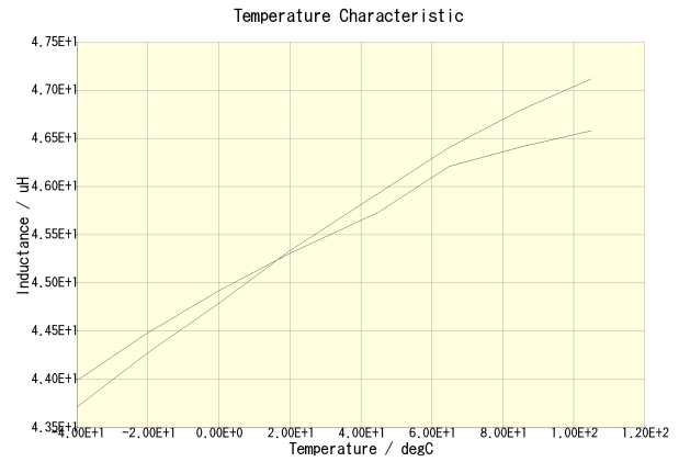
SLF10145T-470M1R4-PF(DC = 0A) SLF10145T-470M1R4-PF(DC = 0.7A)
