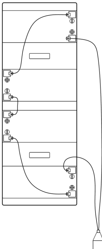
Рисунок 7 — схема соединений АКБ
