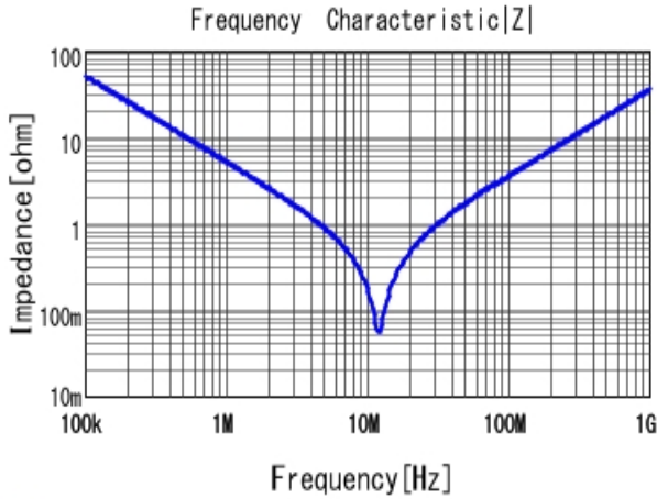
■ RDER72J333K3M1H03A |Z| DCOV, 25degC
