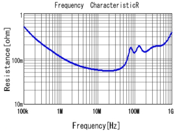
■ RDER72J333K3M1H03A R DCOV, 25degC
