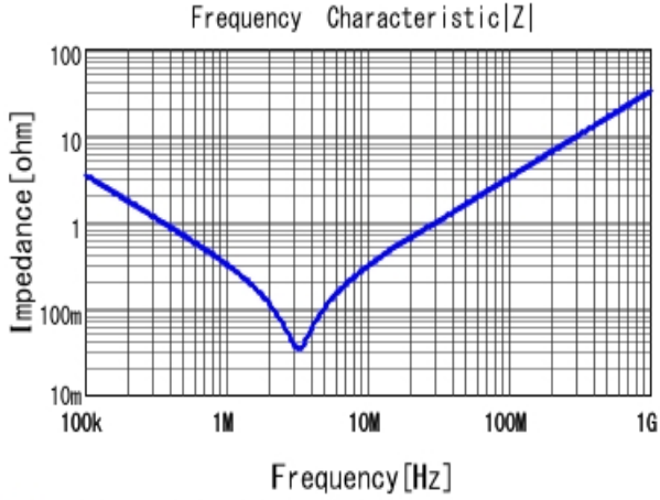
■ RDER71H474K1M1H03A |Z| DC0V, 25degC
