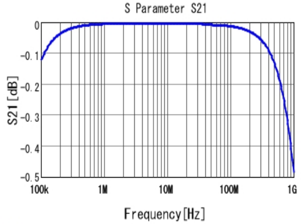
■ RDER71H104K0S1H03A S21 DC0V, 25degC
