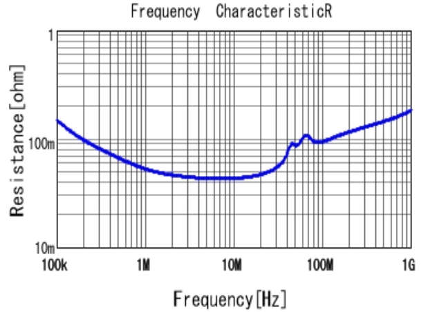
■ RDER71H104K0S1H03A R DC0V, 25degC
