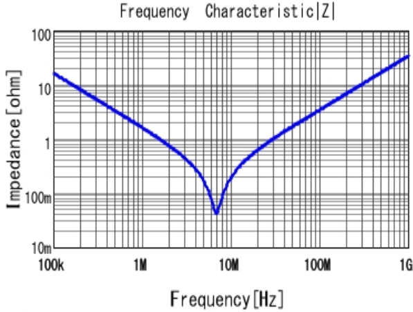
■ RDER71H104K0S1H03A |Z| DC0V, 25degC
