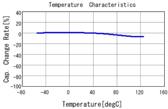
■ RDER71H104K0M1H03A C-Temp. capchange, DC0.0V, AC1.0Vr
