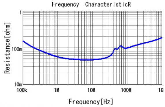
■ RDER71H104K0M1H03A R DC0V, 25degC
