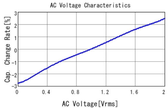
■ RDER71H104K0M1H03A C-AC Voltage capchange, DC0V, 25.0
