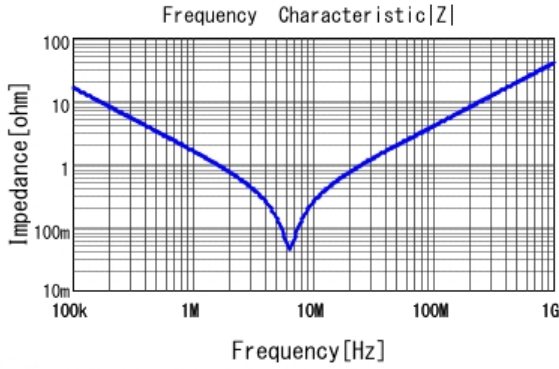
■ RDER71H104K0M1H03A |Z| DC0V, 25degC
