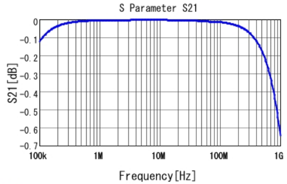
■ RDER71H104K0M1H03A S21 DC0V, 25degC
