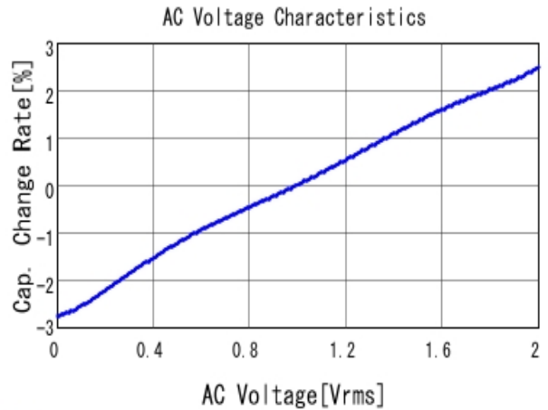
■ RDER71H104K0K1H03B C-AC Voltage capchange, DCOV, 25.0
