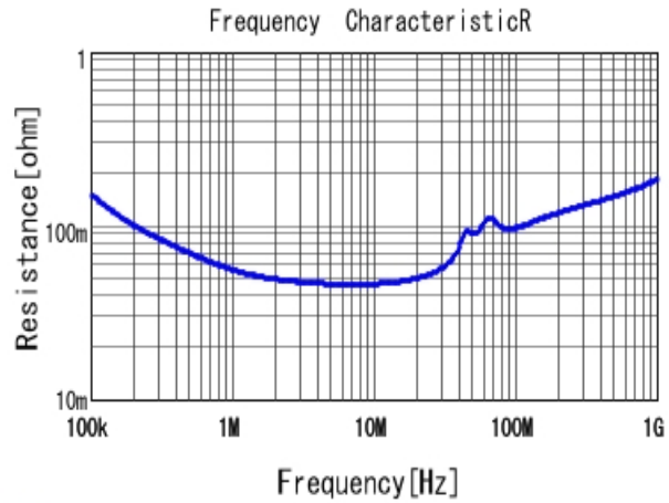
■ RDER71H104K0K1H03B R DCOV, 25degC
