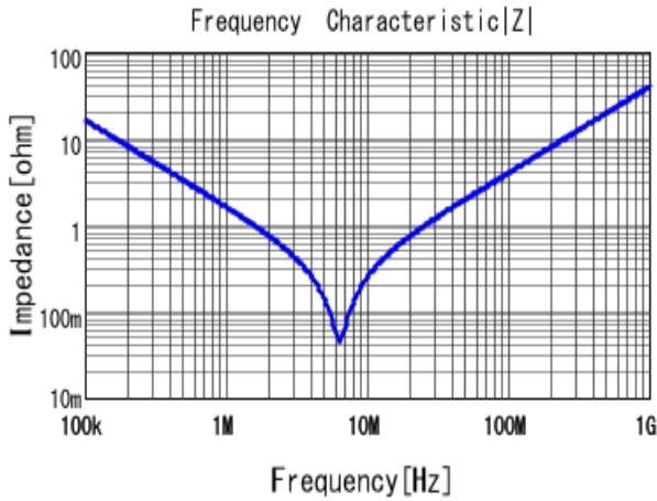
■ RDER71H104K0K1H03B |Z| DCOV, 25degC
