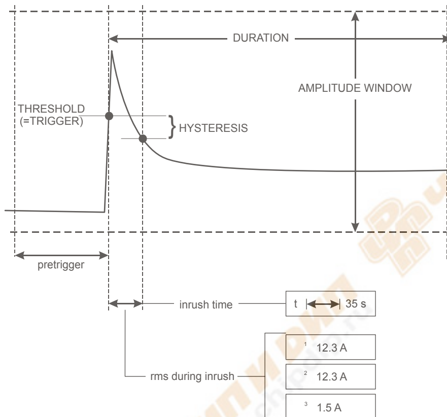
Рис. 15-1 Характеристики пускового броска и соотношение с меню пуска
