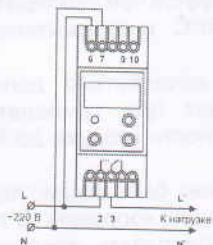
Схема подключения
