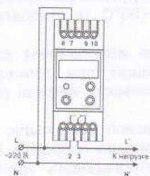
Схема подключения
