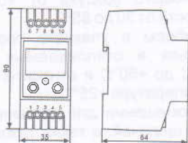
Габаритные размеры
