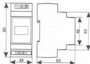
Габаритные размеры
