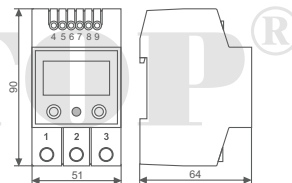
Габаритные размеры
