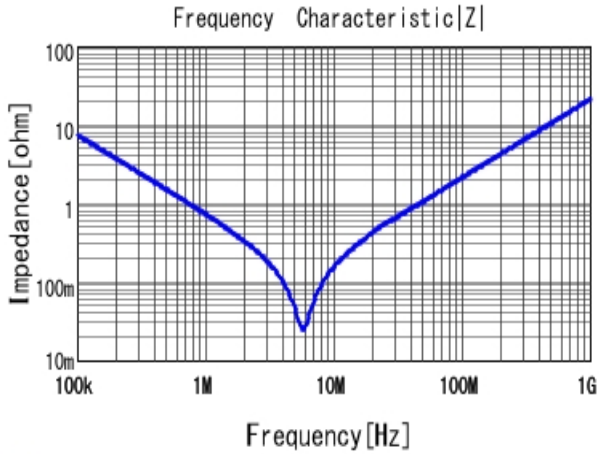
■ RCER71H224K1A2H03B |Z| DCOV, 25degC
