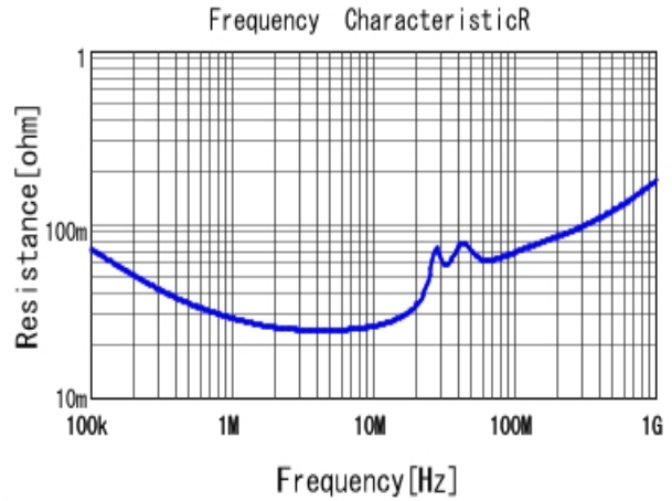
■ RCER71H224K1A2H03B R DCOV, 25degC
