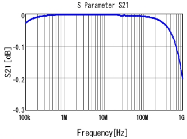
■ RCER71H224K1A2H03B S21 DC0V, 25degC
