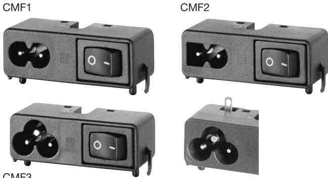
additional ground terminal / zusätzlicher Schutzleiteranschluss
