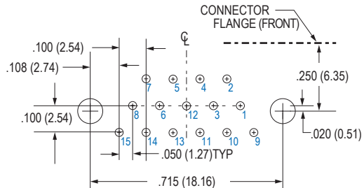
15 SOCKET M83513/13-B
