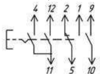
Электрическая схема коммутации
