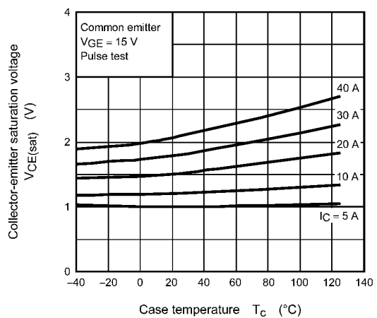
Fig. 8.6 V_{CE(sat)} - T_C
