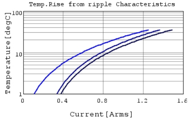
GRT155R71C104KE01 Temp.rise — 400kHz —
