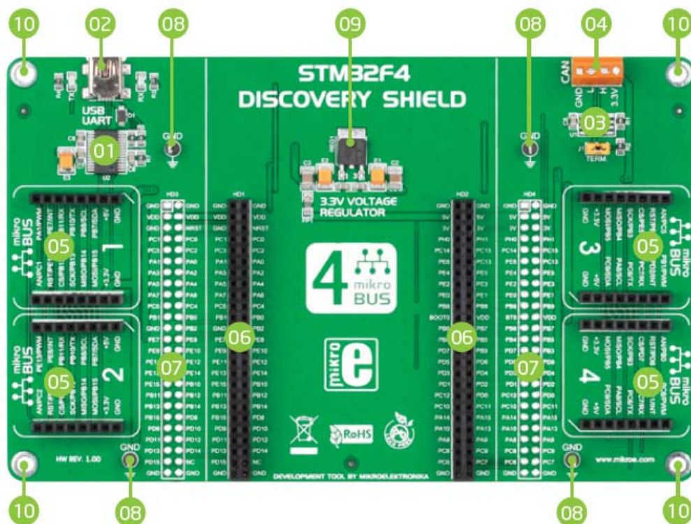
Рисунок 1-1: STM32F4 Discovery shield
