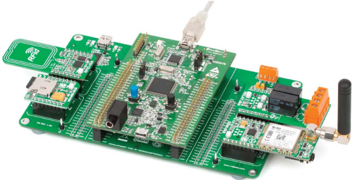
Рисунок 1-2: STM32F4 Discovery плата подключена к четырем Click платам через модуль STM32 Discovery Shield
