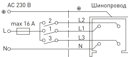
а) 1 фаза, 3 нагрузки, АС 230 В, 16 А, 3,7 кВА
