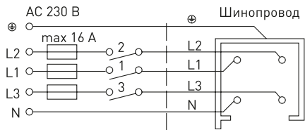
б) 3 фазы, 3 нагрузки, АС 230 В, 16 А, 3×3,7 кВА
