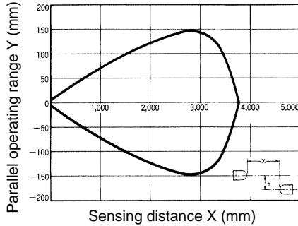
E32-T14 with E3X-NH amplifier
