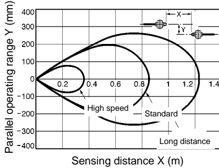
E32-T11R with E3X-DA amplifier
