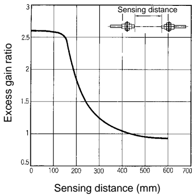
E32-TC200 with E3X-NM and E3X-NT amplifiers
