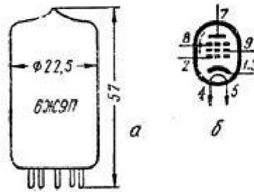
Лампа 6Ж9П:
