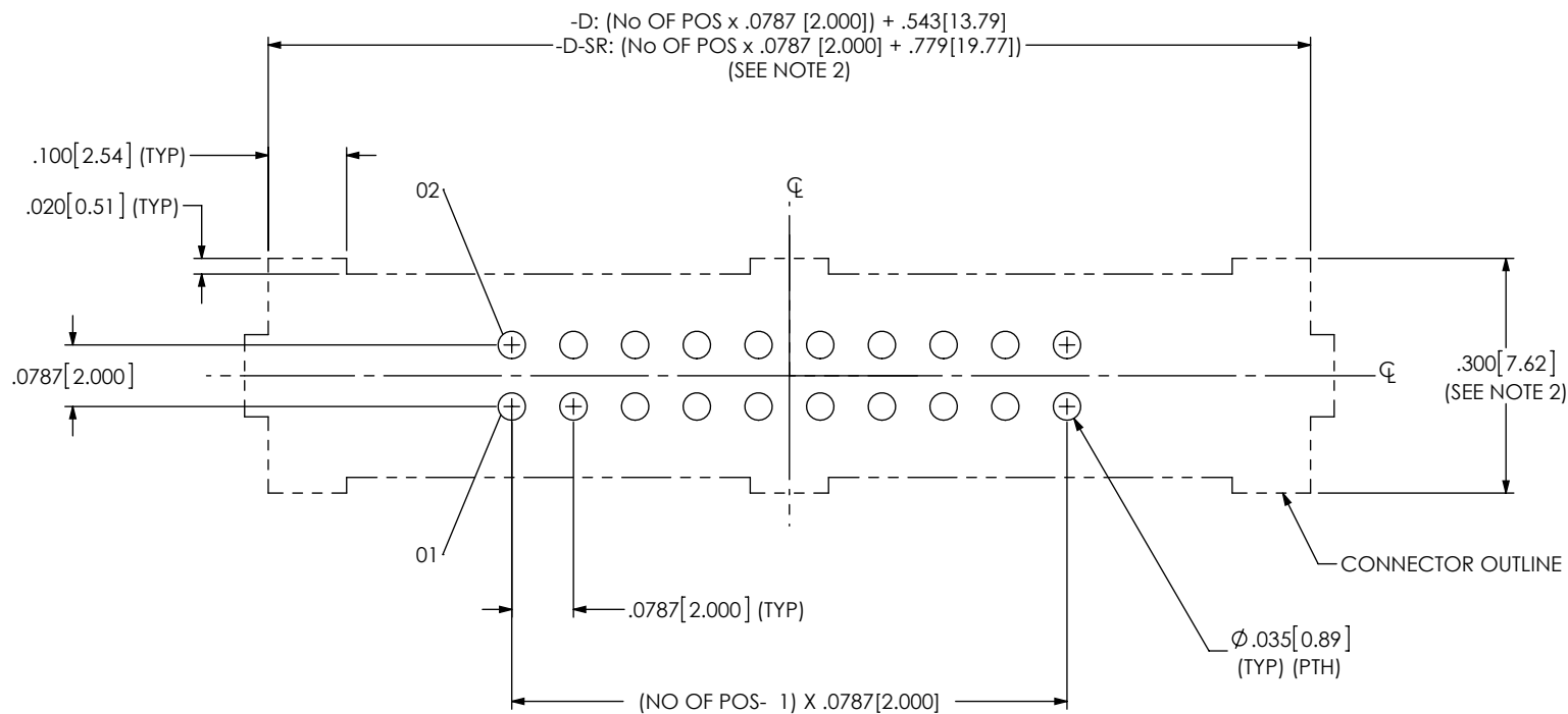
FIG 4 EHT-110-01-X-D & EHT-TT0-01-X-D-SR SHOWN
