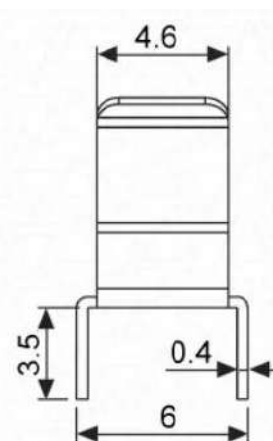
Артикул Q-2642a покрытие – Ag
