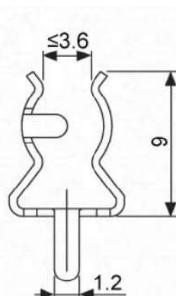
Артикул Q-2642a покрытие – Ag
