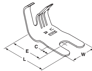
B Tab-Lok
