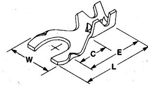
B SPADE-LOK
