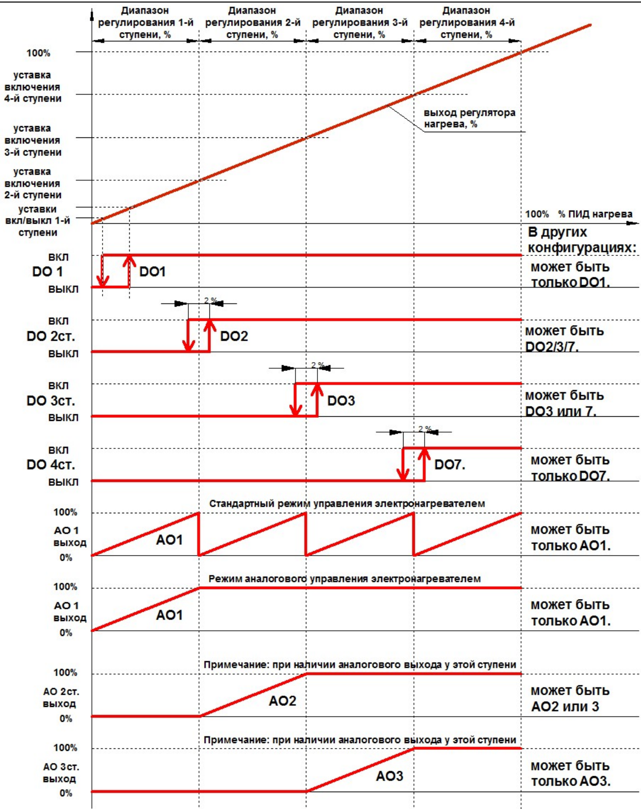
рис. 2. Логика работы 4-хступенчатого электронагревателя.
