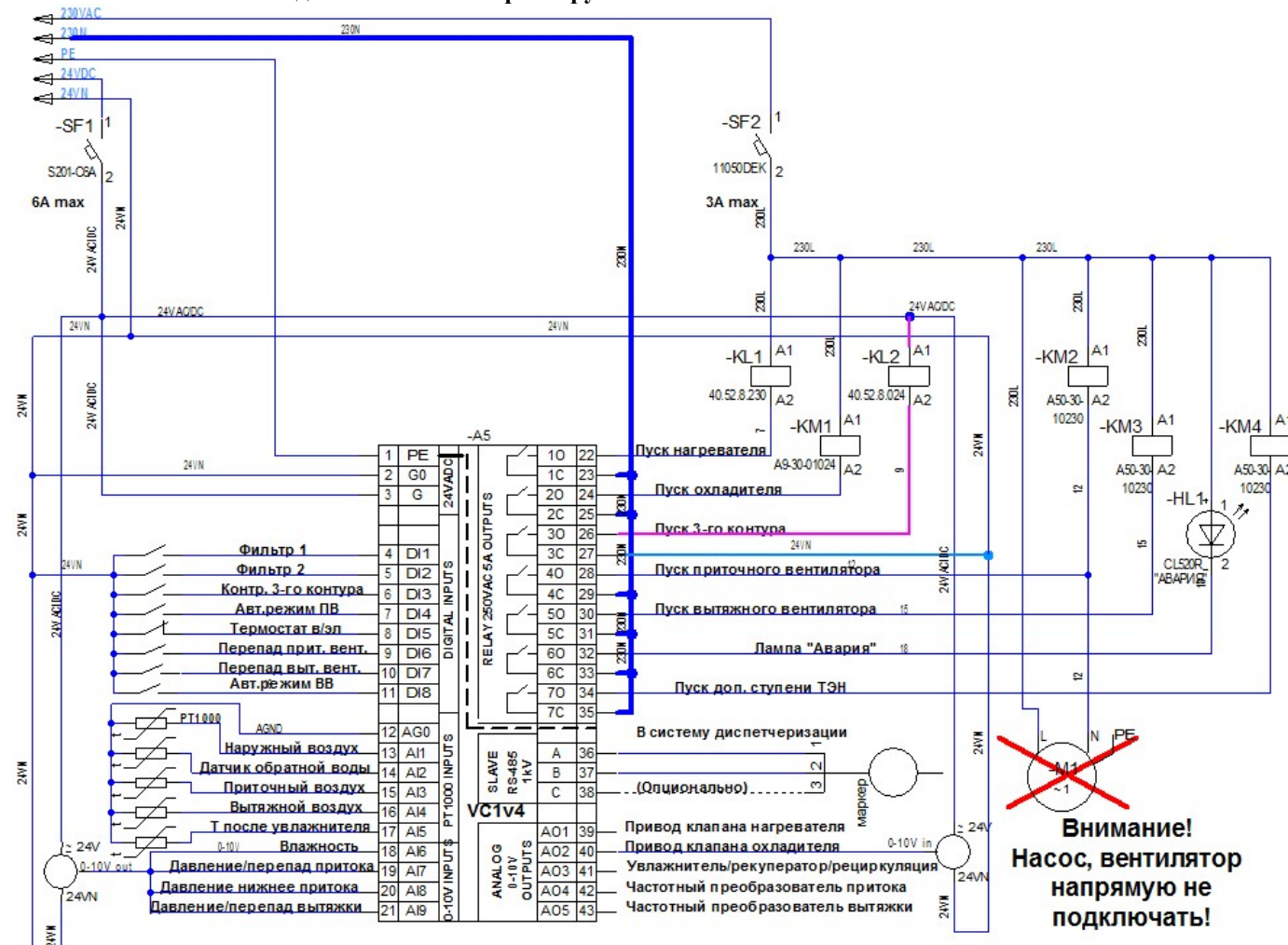
Рис.1а Схема внешних подключений к контроллеру VC1.
